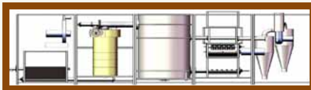
Страничен поглед на електроцентралата
